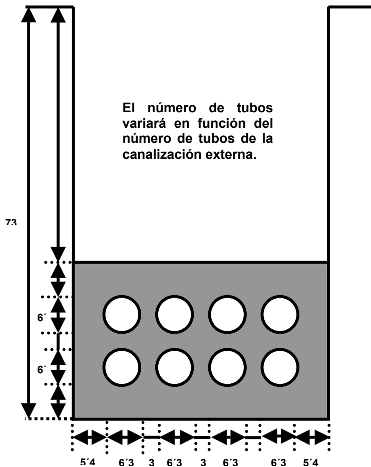
APÉNDICE 4: EJEMPLO DE SECCIÓN TRANSVERSAL DE CANALIZACIÓN DE ENLACE SUBTERRANEA DE 8 TUBOS.
